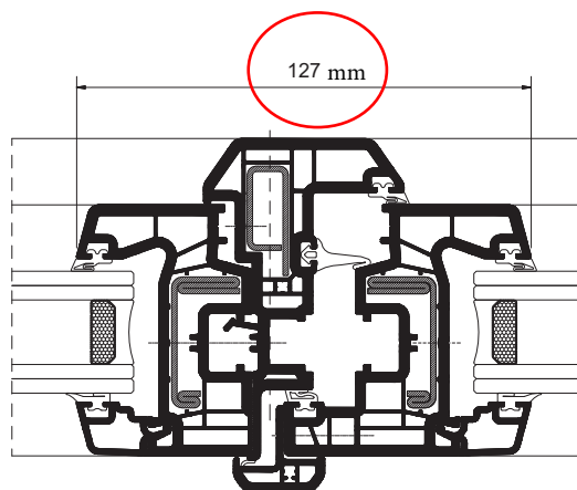
Nudo central A 70 Abisagrada triple junta
