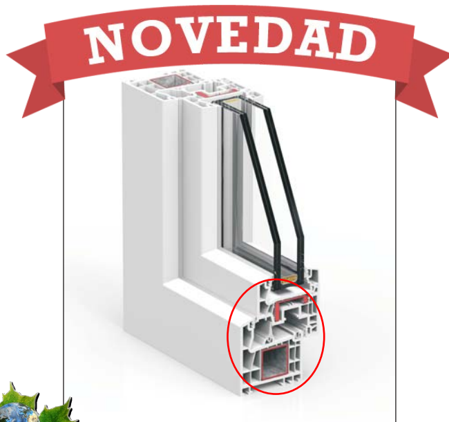
Nudo central A 70 Abisagrada triple junta
